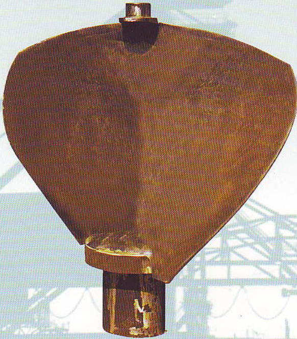
PALES D'HÉLICES À PAS VARIABLE JUSQU'À 1500 KG
